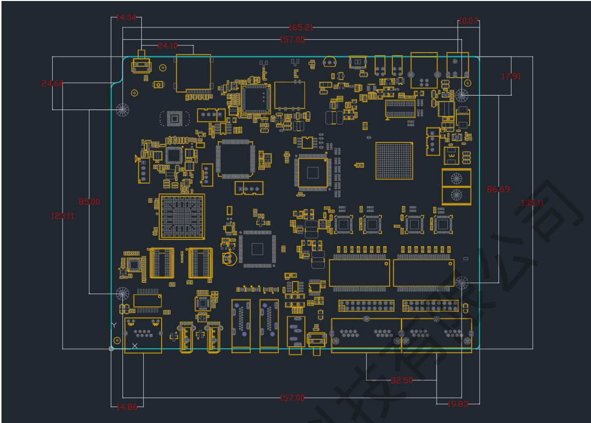
M80 裸卡尺寸图
