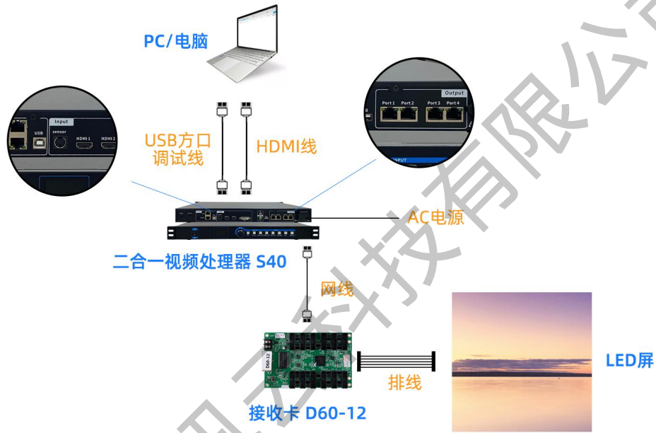
S40 硬件连接图
