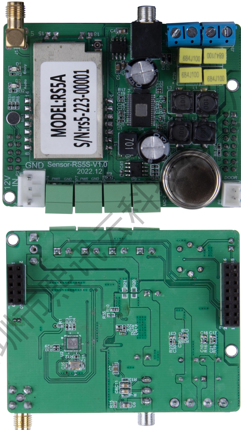
Lora 无线同步模块多功能卡 RS5A
