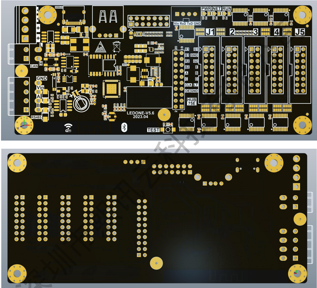
控制卡 3D
