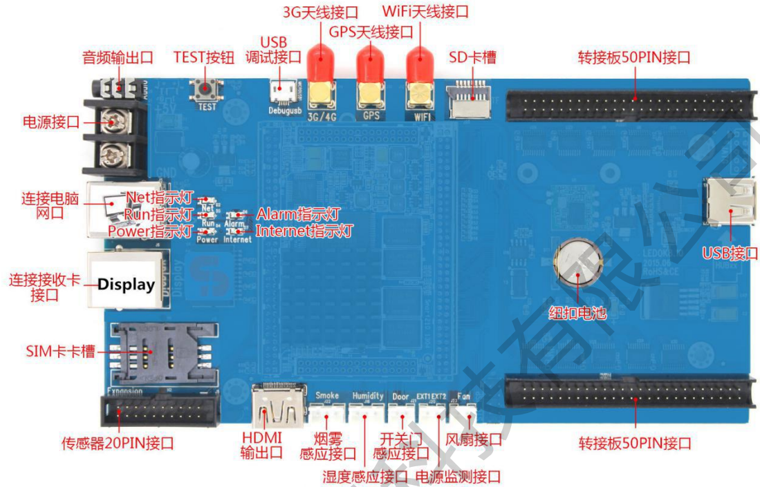
Y10 接口示意图
