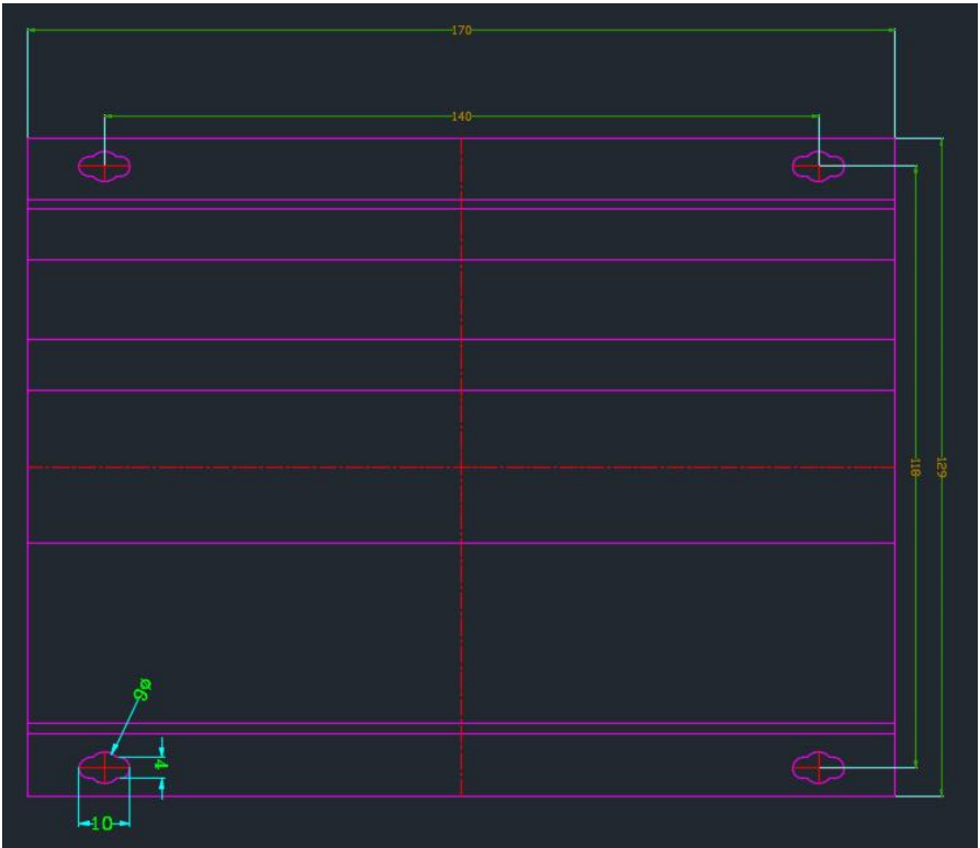
控制盒 M70B-L 安装尺寸图
